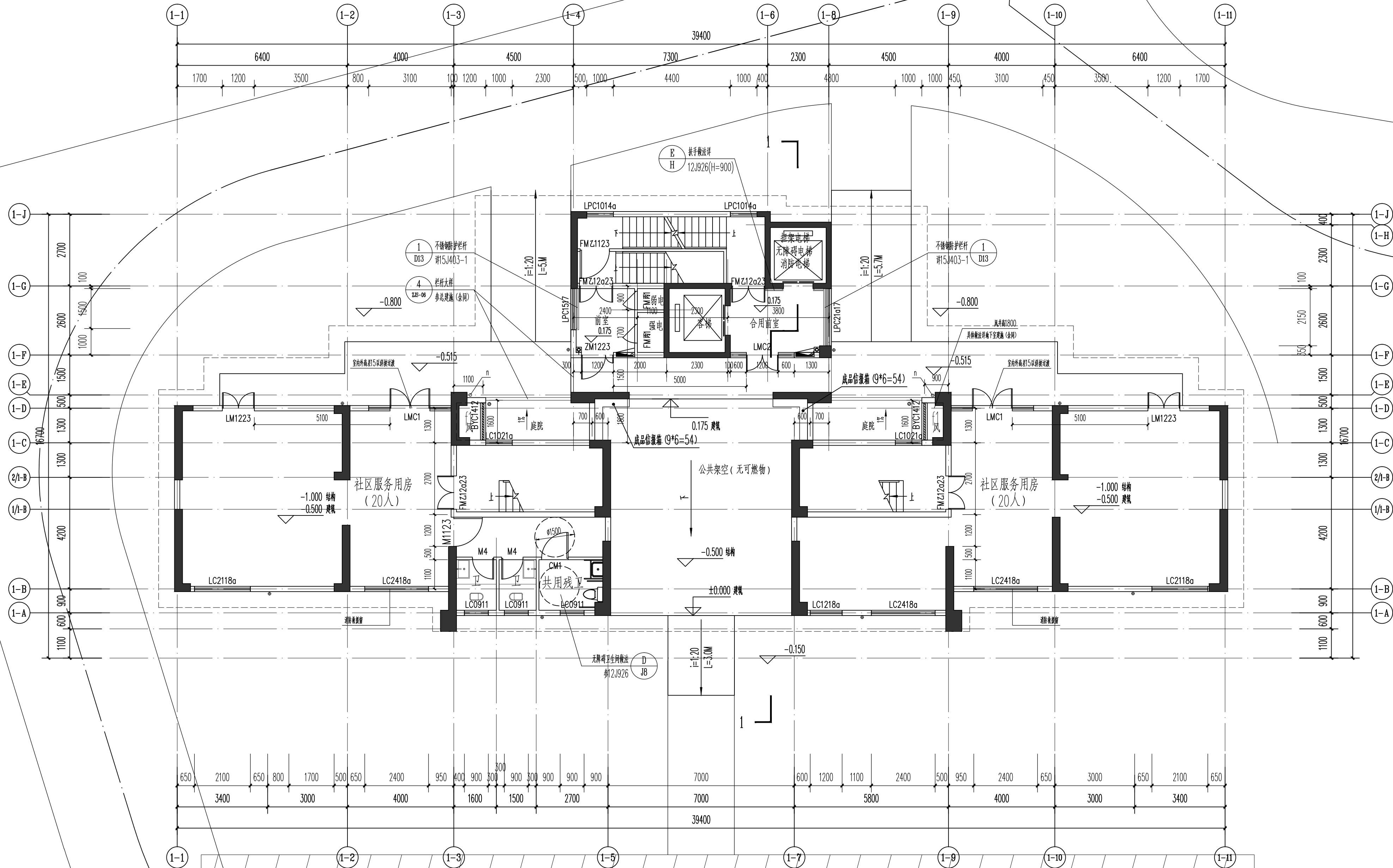
一层平面图 1:100
