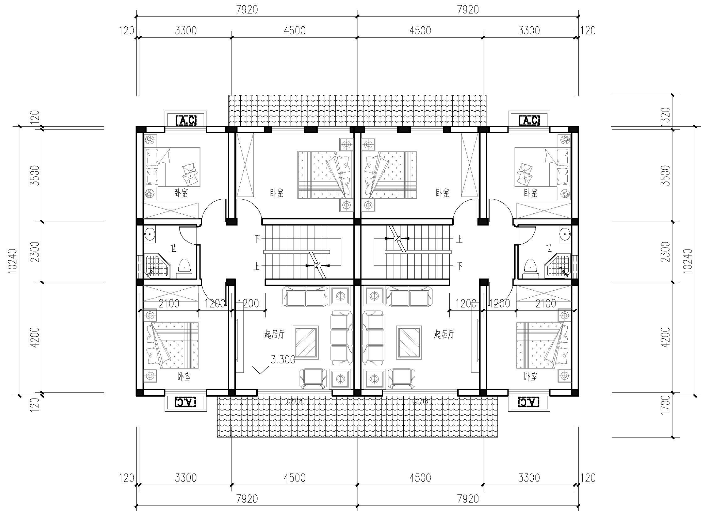
二层平面图
