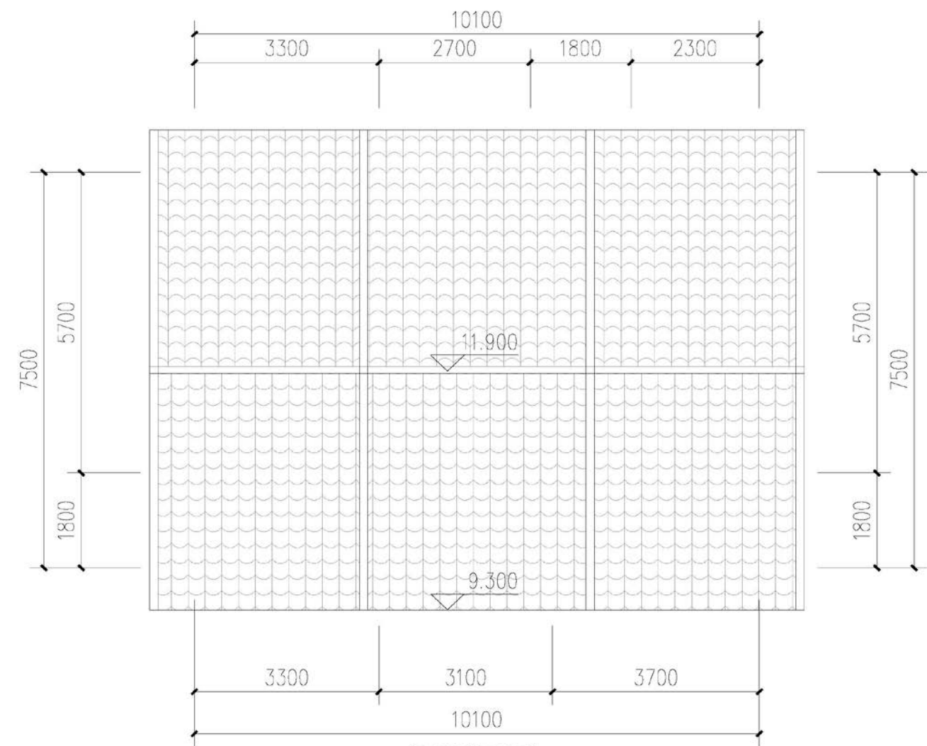
屋面平面图 1:100
