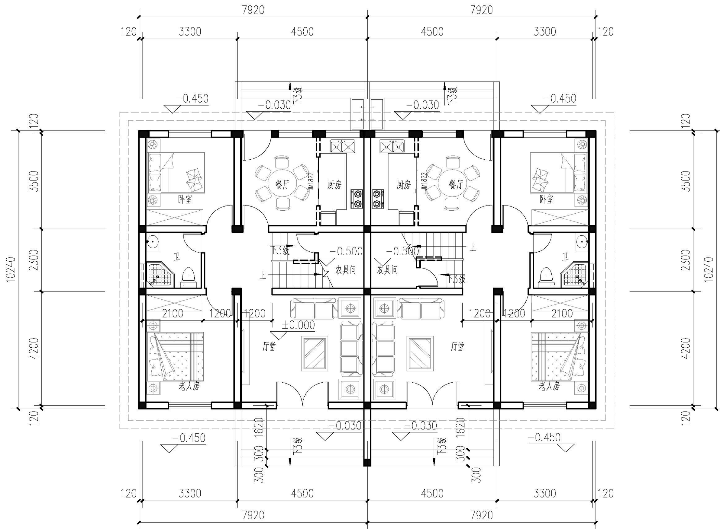
一层平面图
