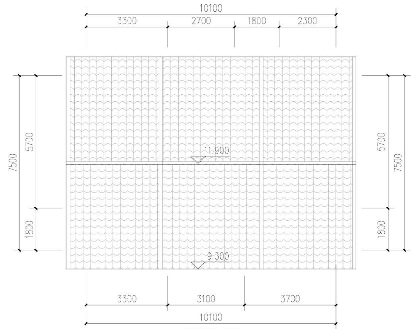
屋面平面图 1:100
