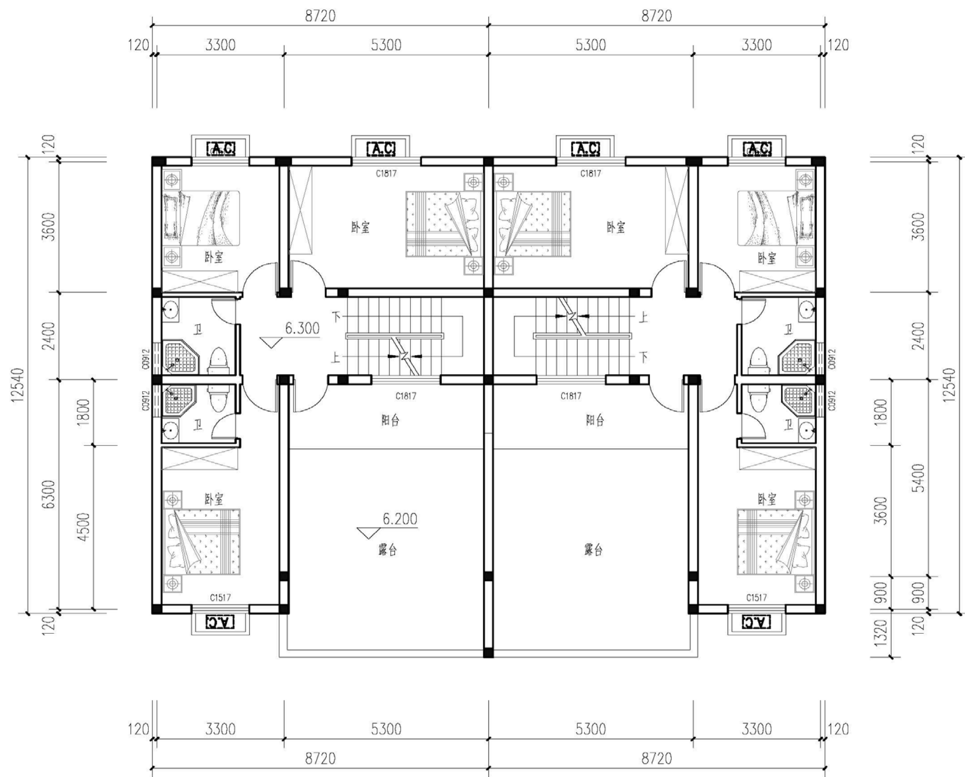
三层平面图
