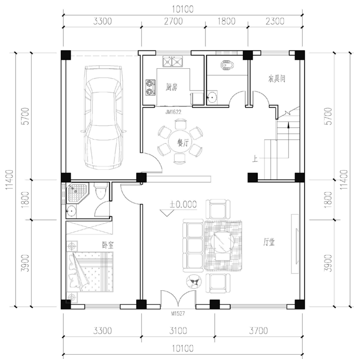
一层平面图
