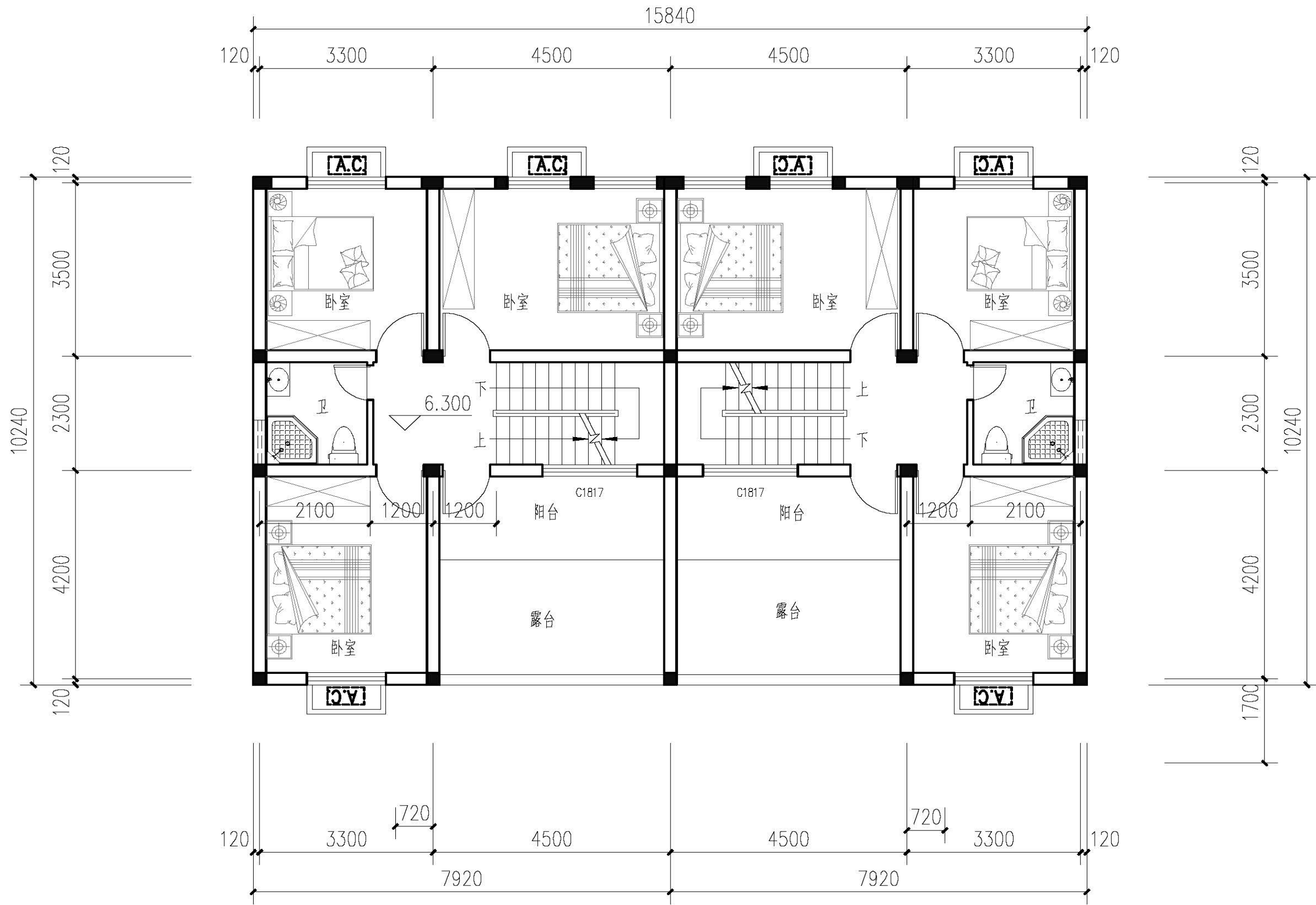
三层平面图
