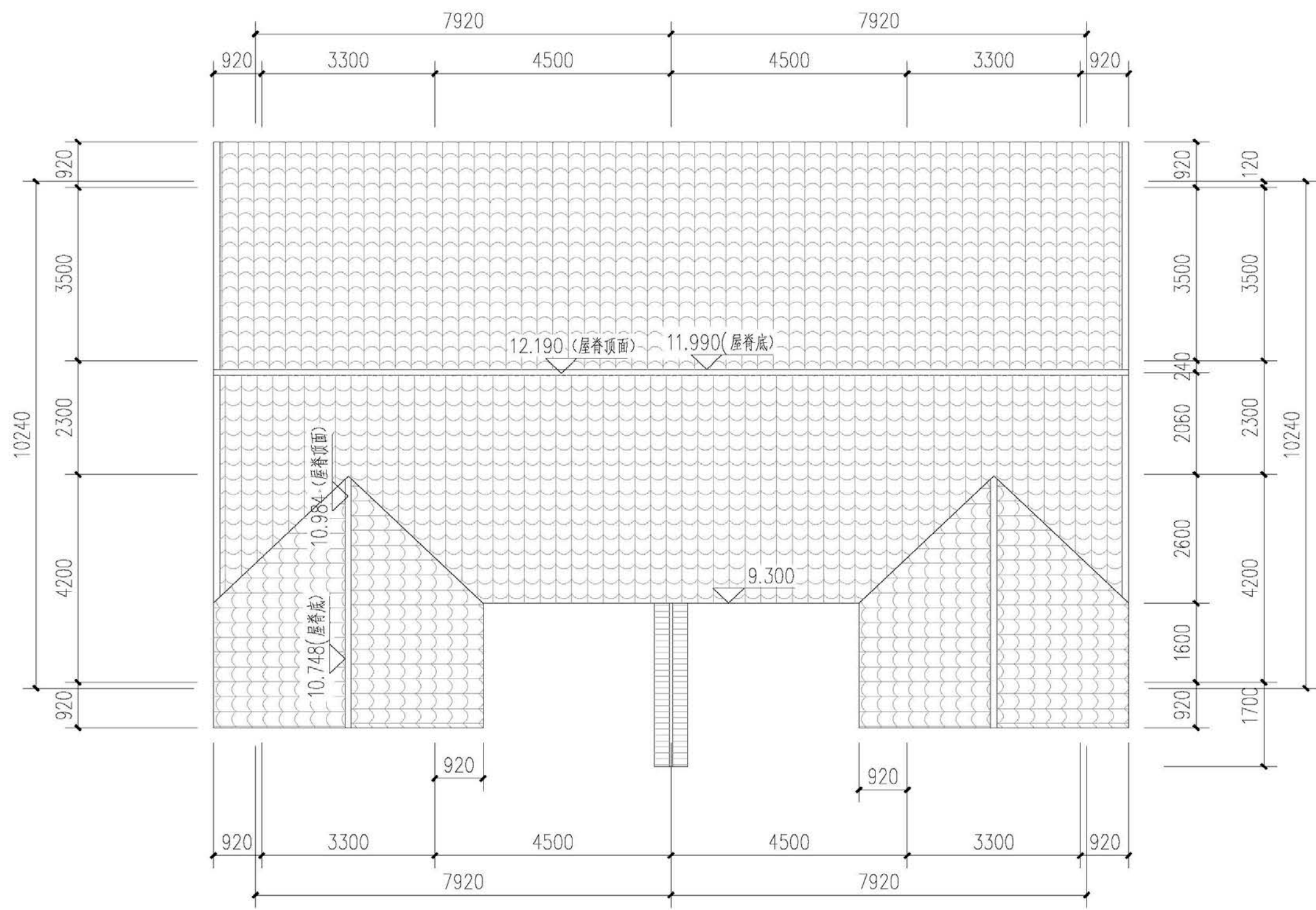
屋面平面图
