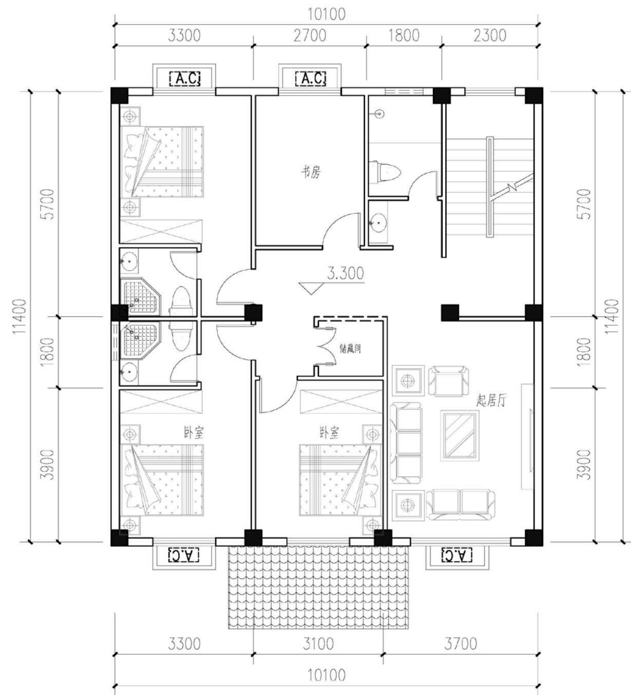
二层平面图
