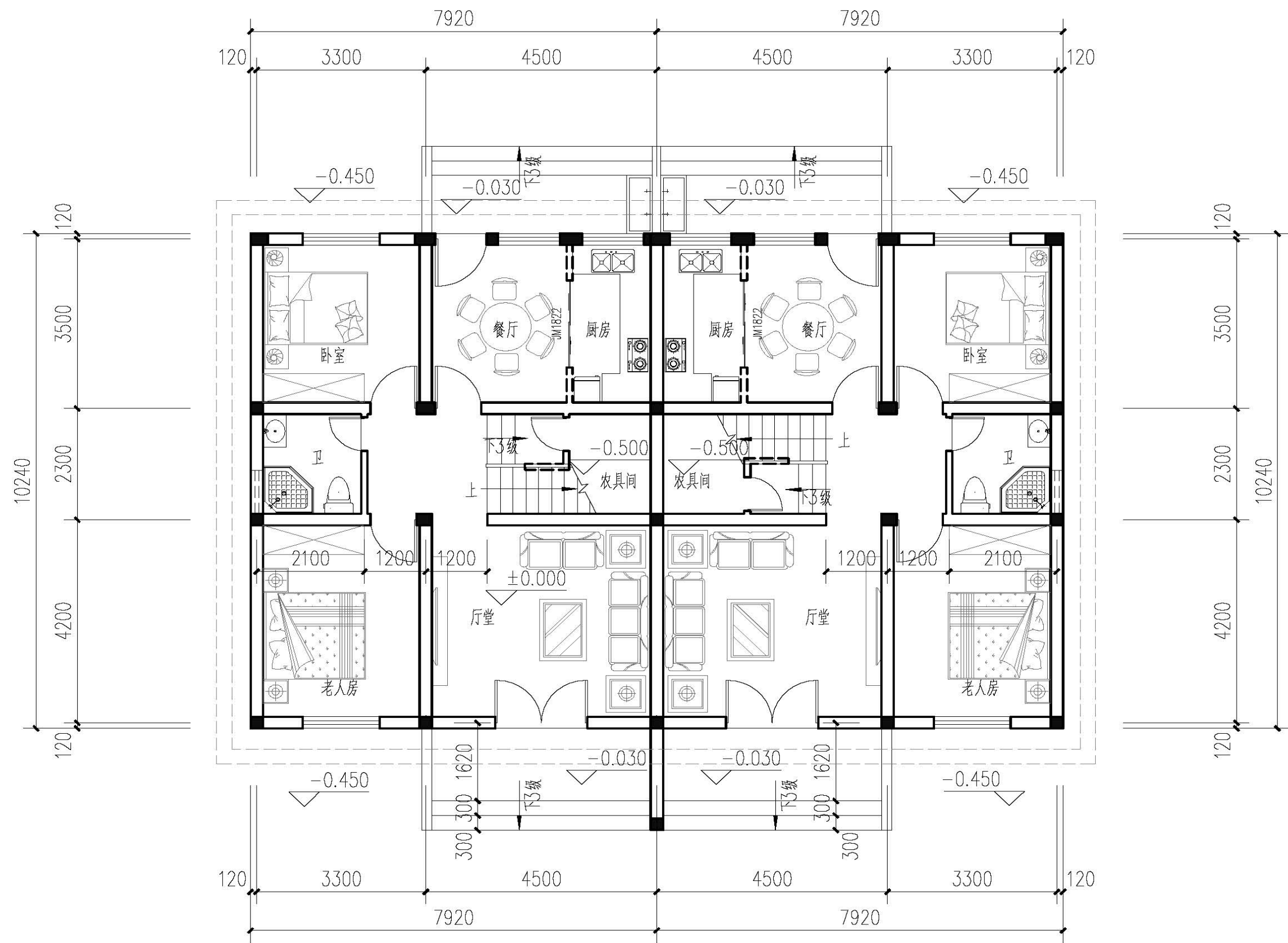
一层平面图
