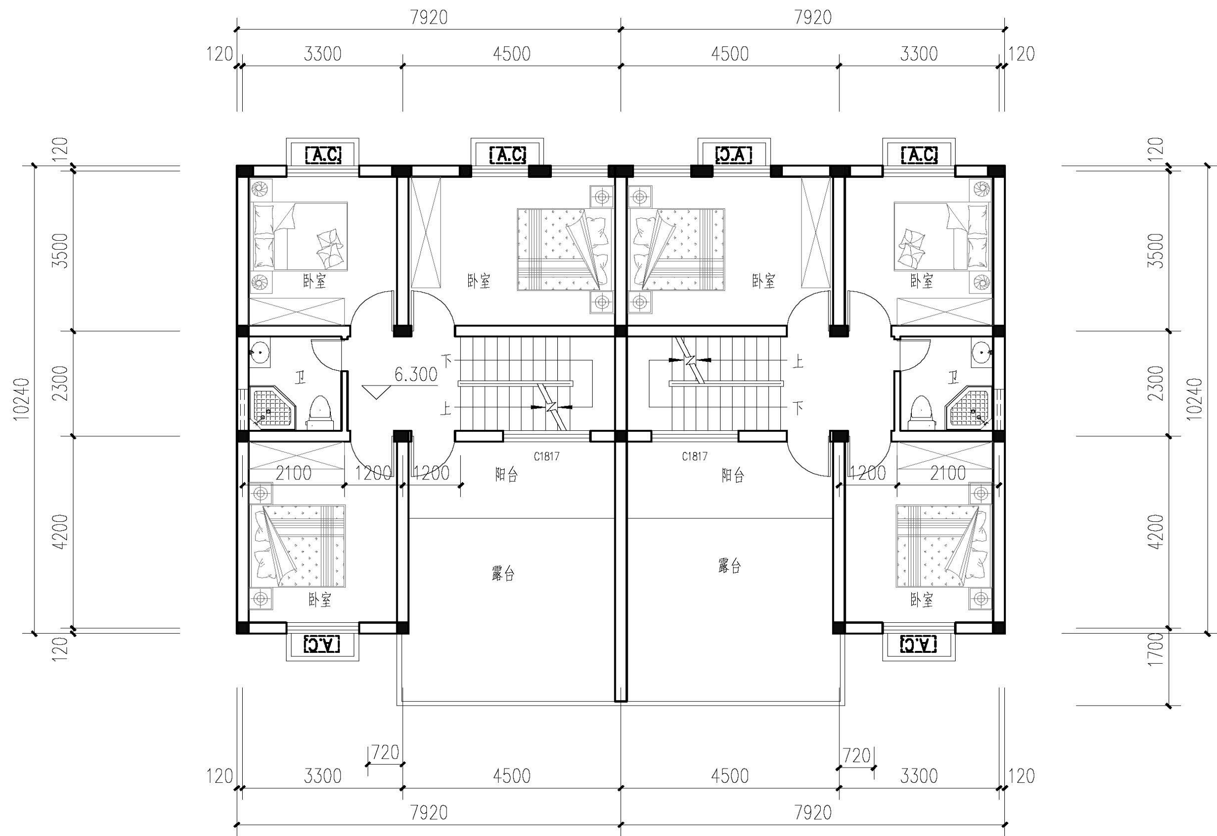
三层平面图
