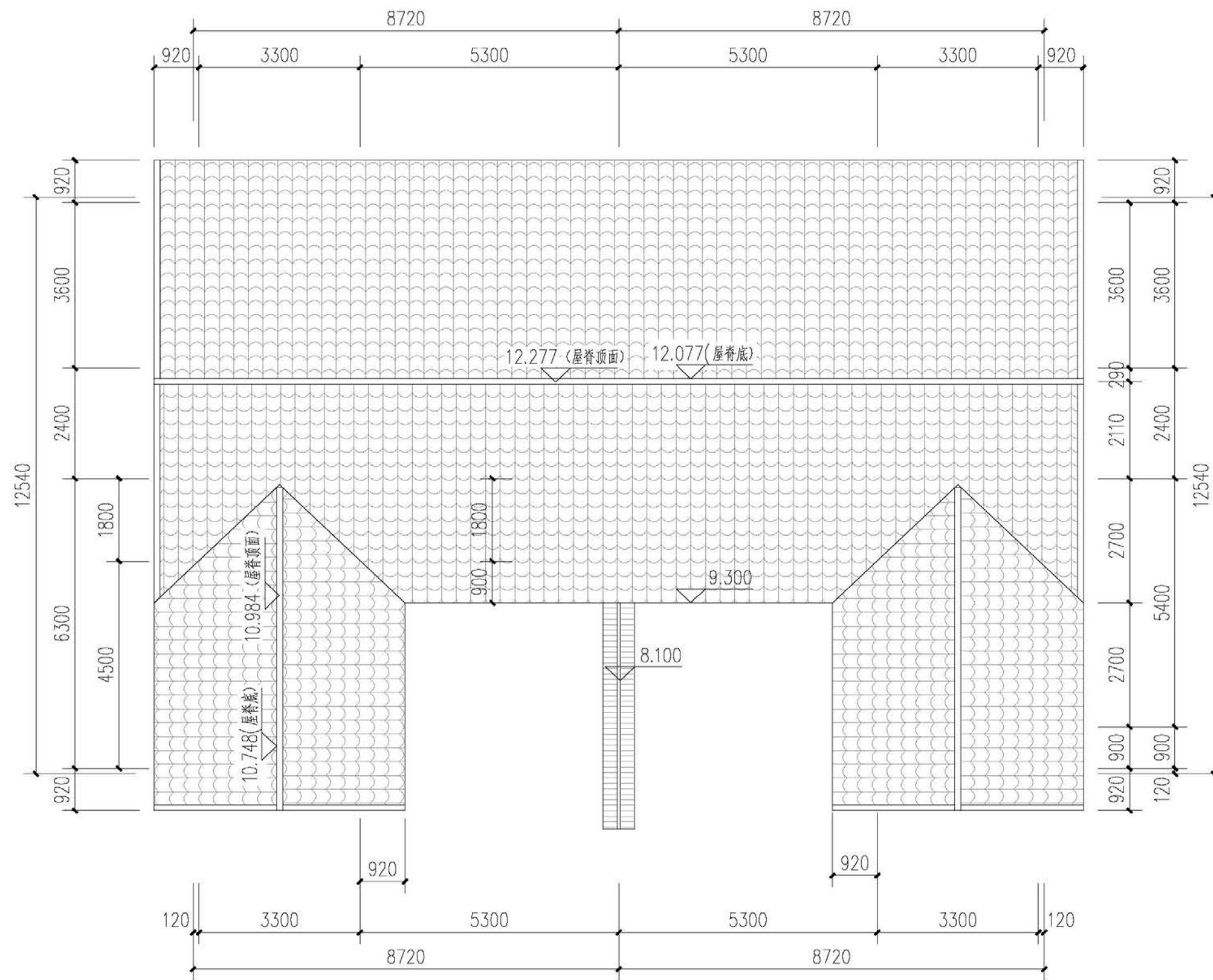
屋面平面图
