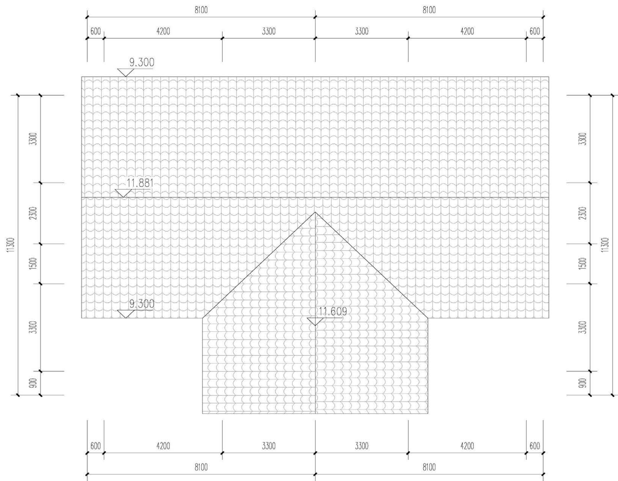
屋面平面图
