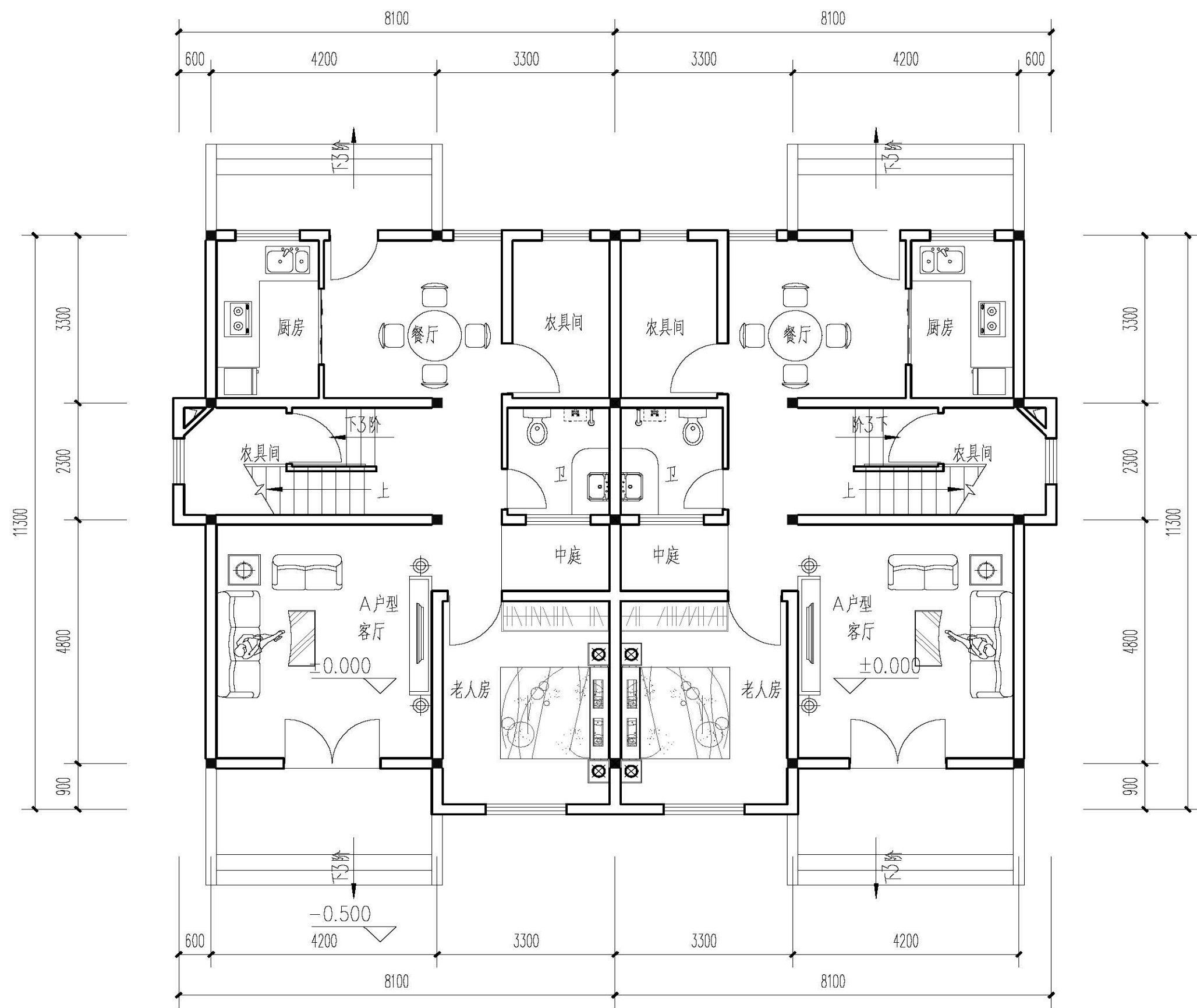
一层平面图
