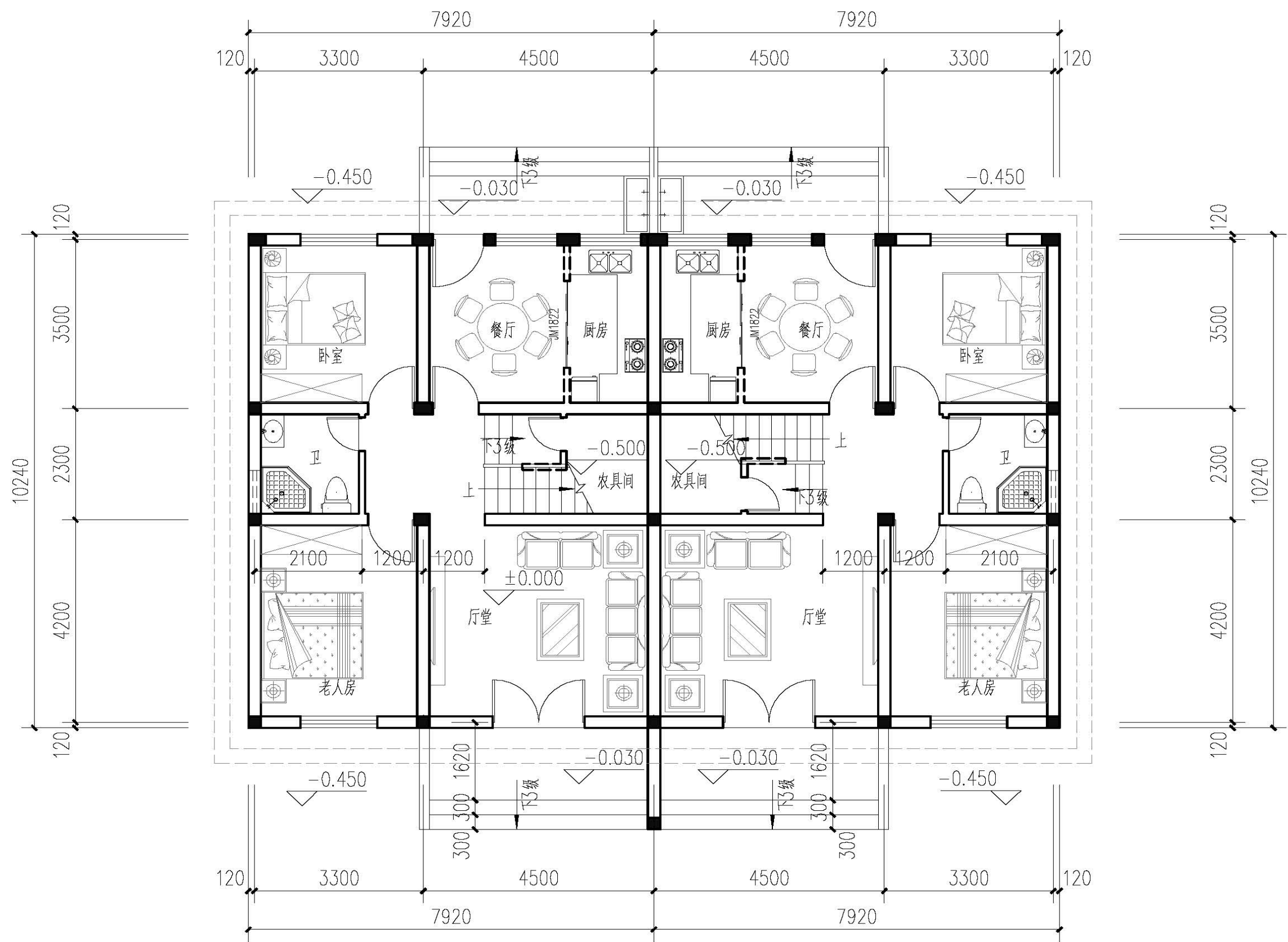
一层平面图
