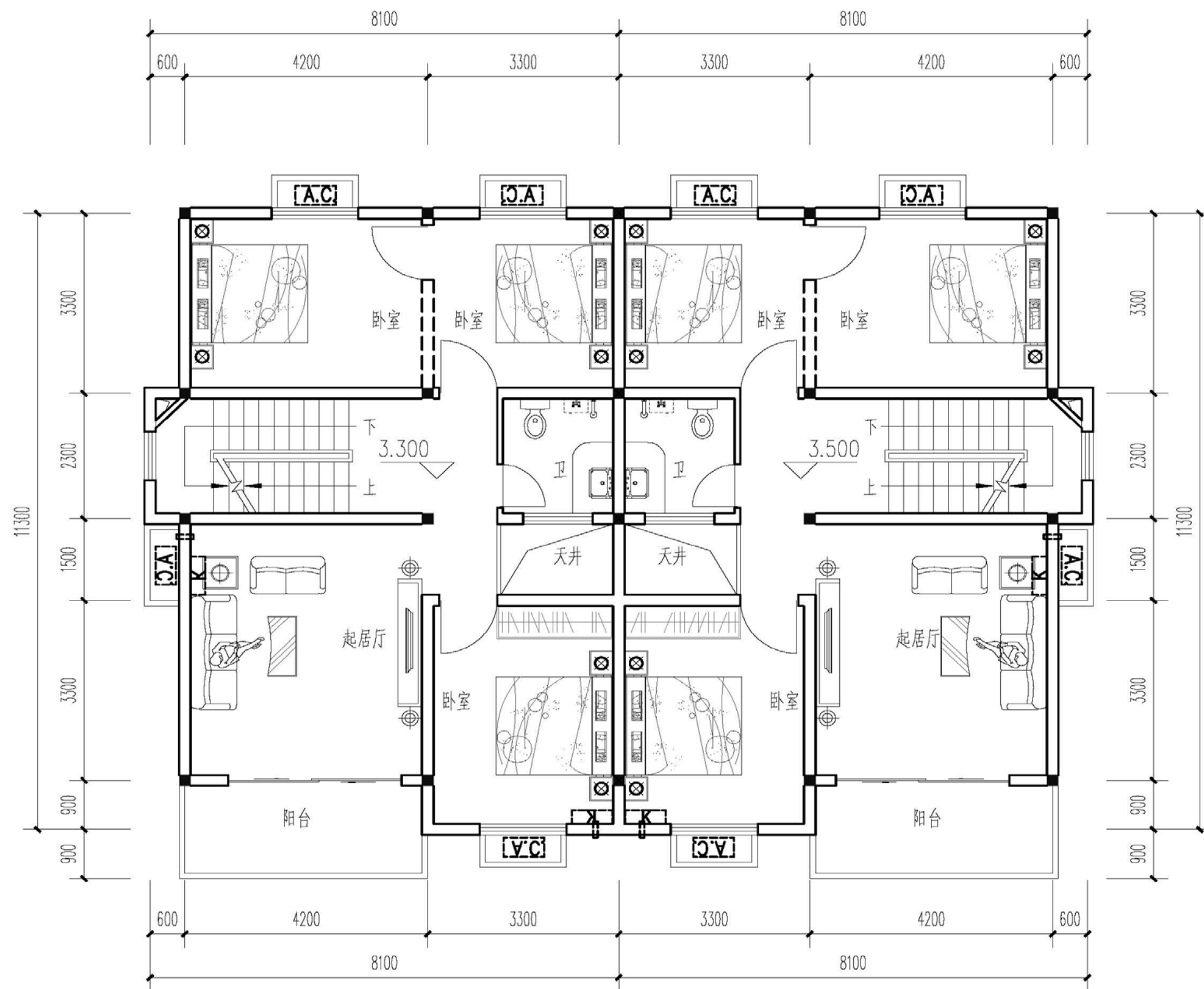
二层平面图
