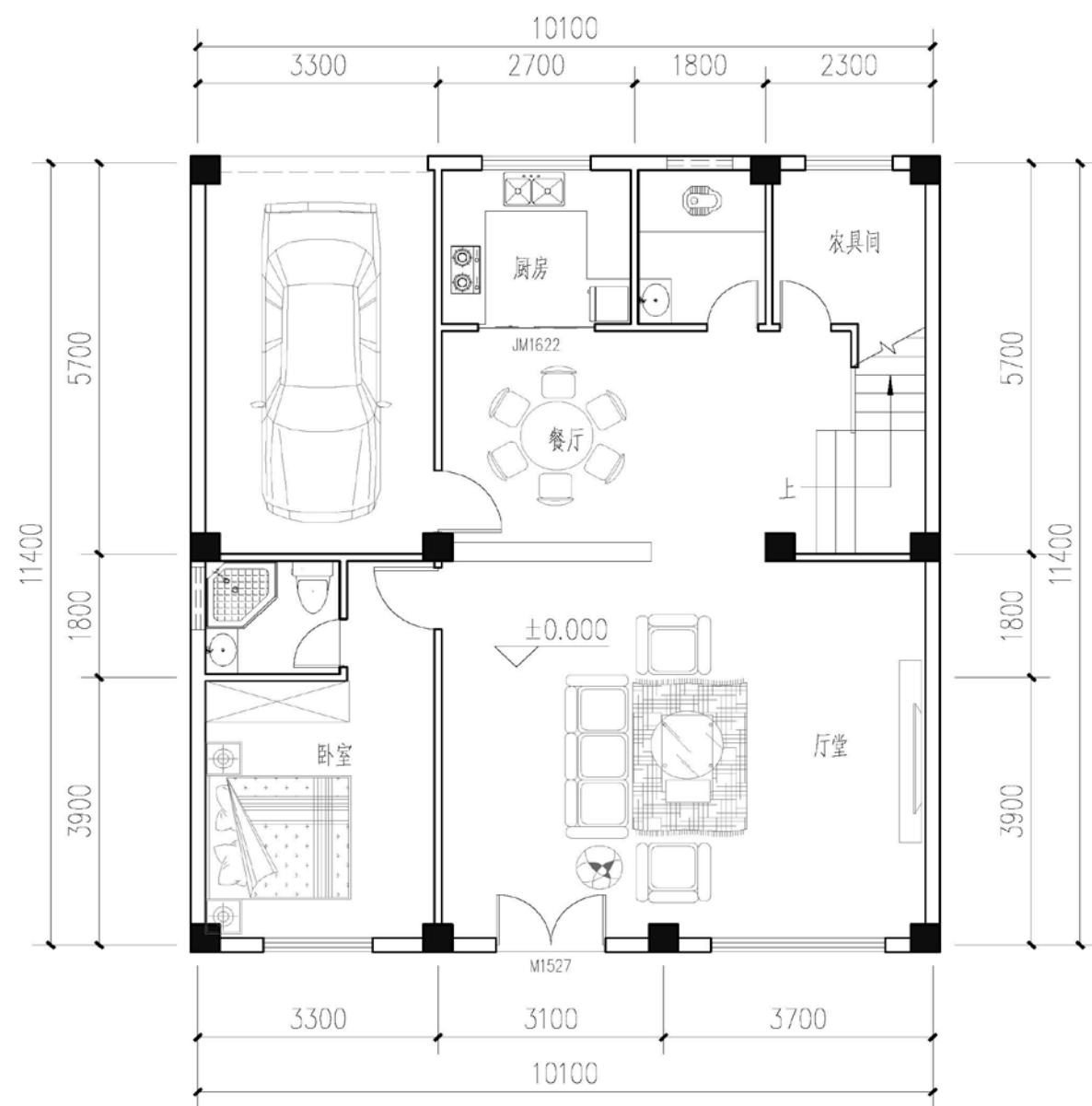
一层平面图
