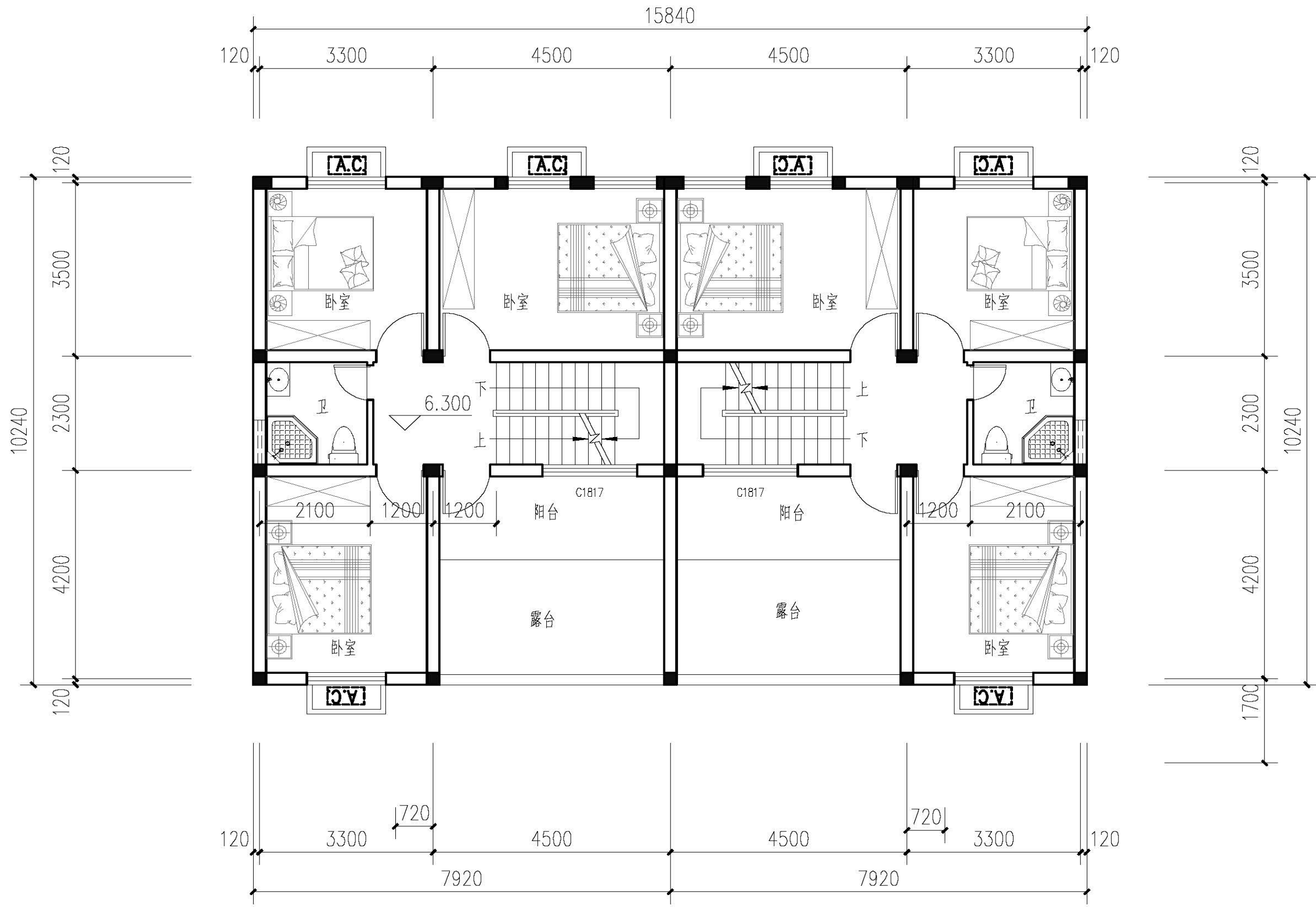
三层平面图
