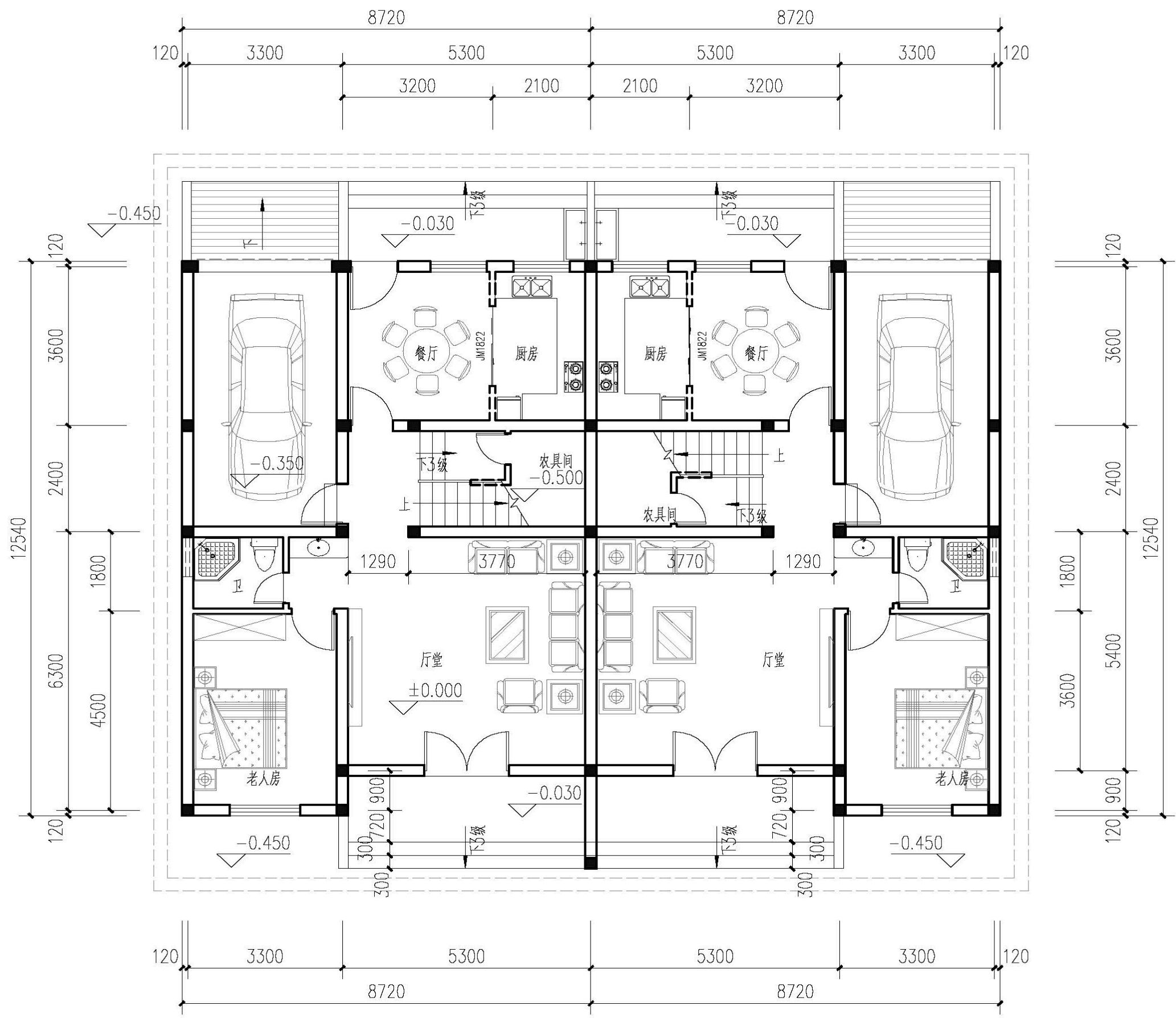
一层平面图
