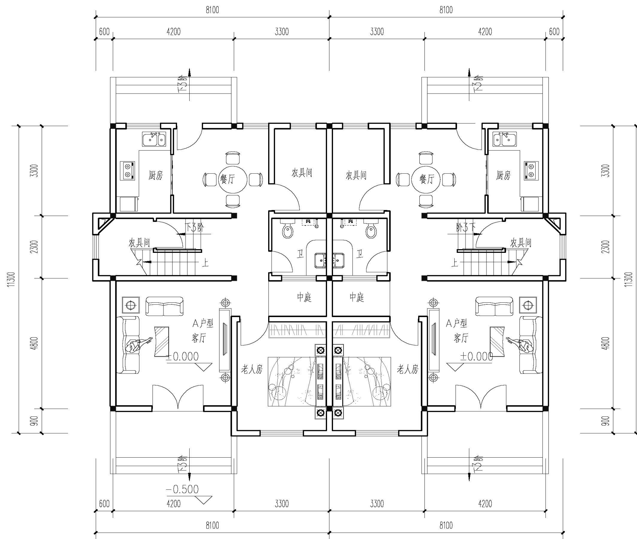
一层平面图
