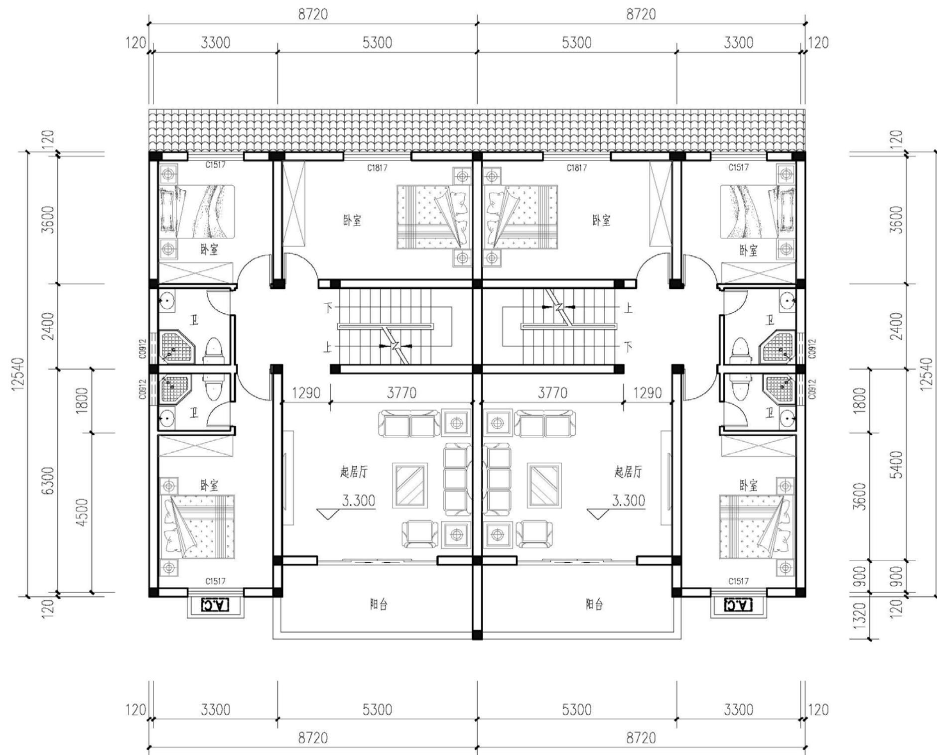
二层平面图
